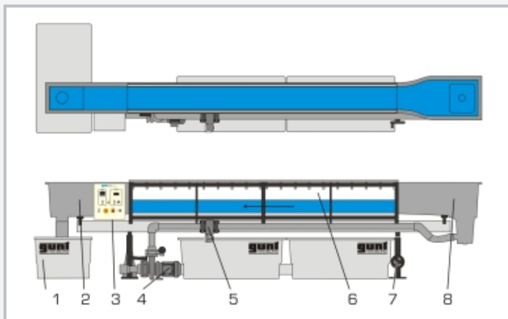
1 depósito de agua, 2 elemento de salida, 3 caja de distribución, 4 bomba, 5 sensor de caudal, 6 sección de ensayo, 7 ajuste de la inclinación, 8 elemento de entrada
