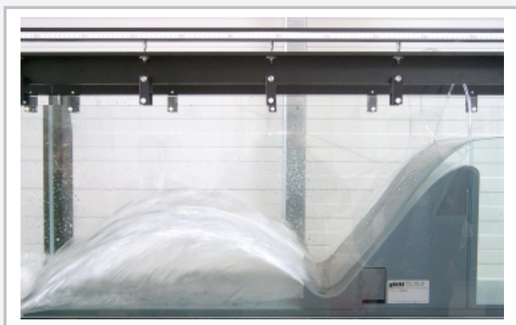
Desbordamiento en presa-vertedero de perfil Oggee con salto de esquí HM 163.32.
