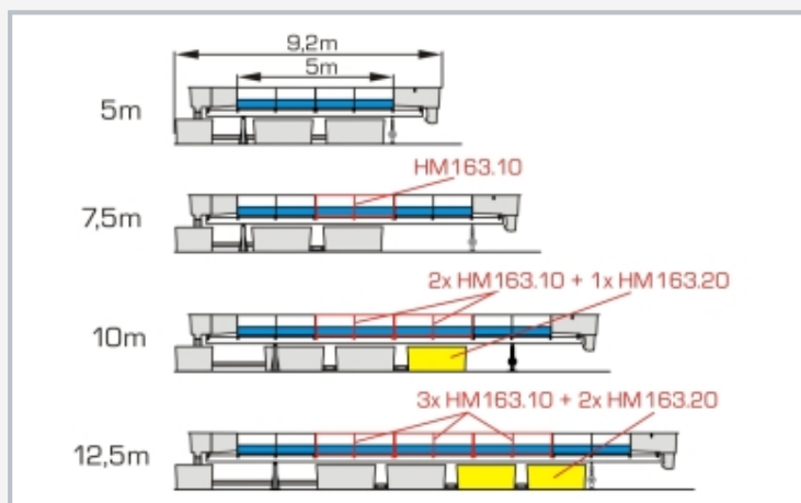
HM 163 con secciones de ensayo de longitudes diferentes (5...12,5m). Dependiendo de la longitud deseada se necesitan también elementos de prolongación adicionales del canal de ensayo HM 163.10 y depósitos de agua HM 163.20.
