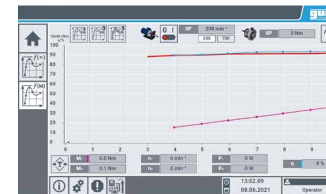
M = 4 - 10 Nm, n = 200 min -1 = const curvas superiores, en rojo: valor nominal de la curva de rendimiento, azul: valor real de la curva de rendimiento
