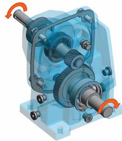
MT120 Kit de montaje: engranaje recto
