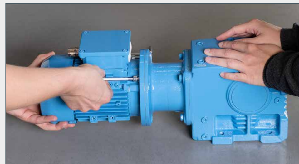
desmonte la cadena de transmisión
